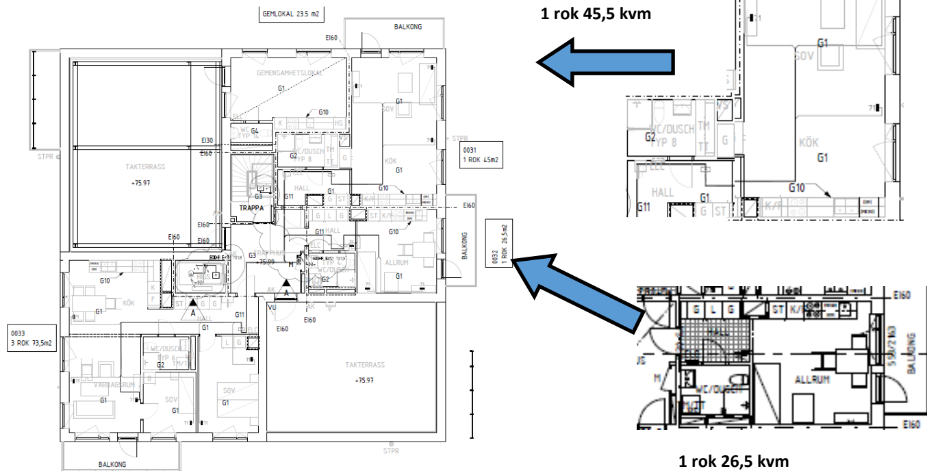
Situationsplan våning 7 med takterasser
